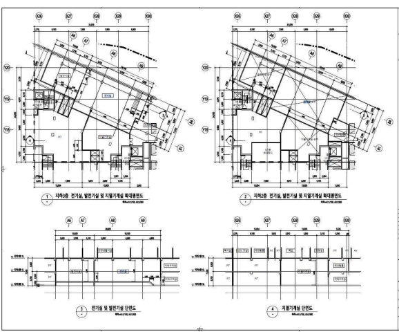
전기실·발전기실·기계실 평·단면도
