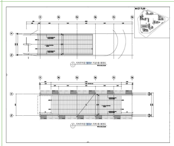
램프 평·단면도
