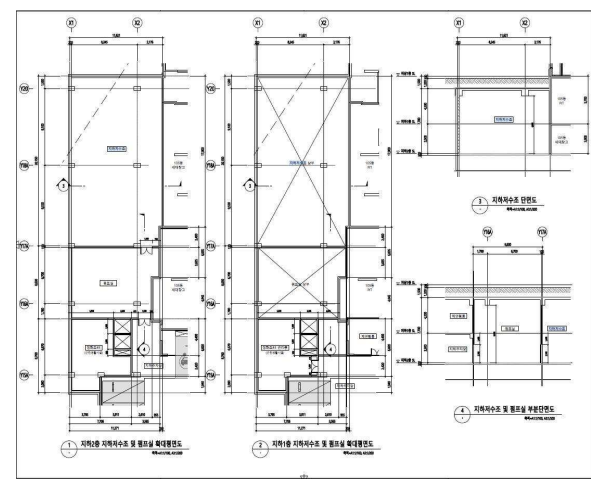
지하저수조 및 펌프실 평·단면도
